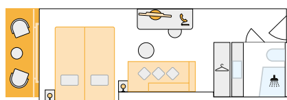
C 2-Bett-Außenkabine mit Balkon, 21 m 2 , auf Deck 2 und 3
